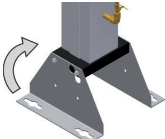
Alésages sur les profilés de pied
