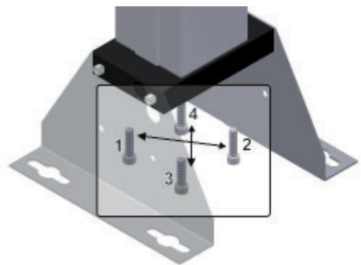
Refixer correctement la plaque inférieure
