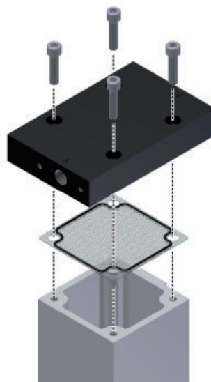
Dévisser la plaque supérieure
