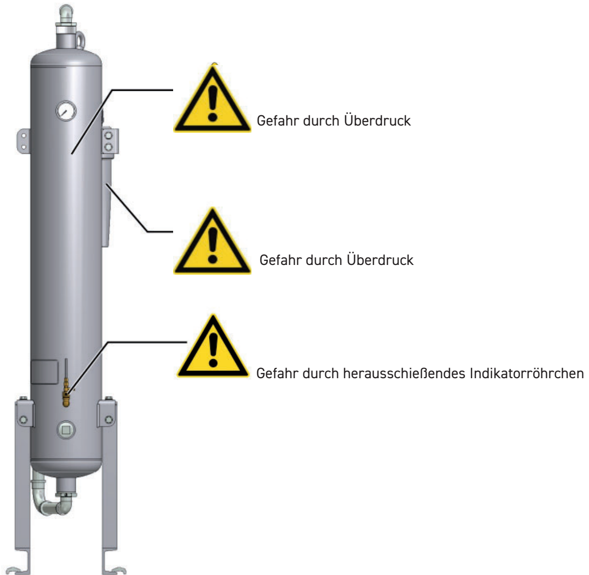
Vorderansicht
