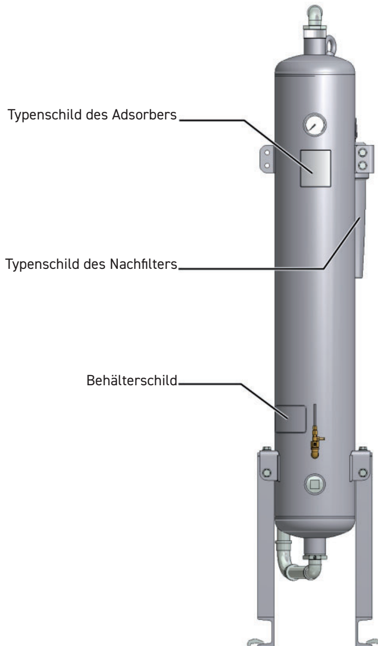
Vorderansicht
